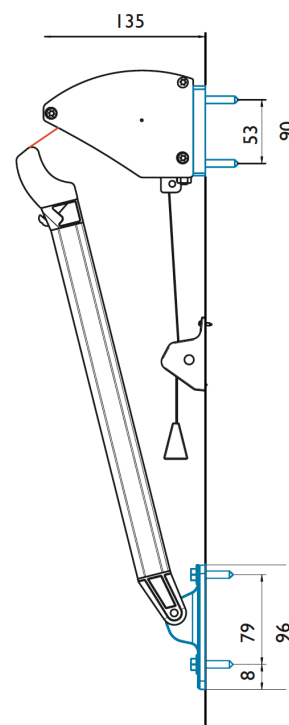
Väggmontering DA32 (mm).
